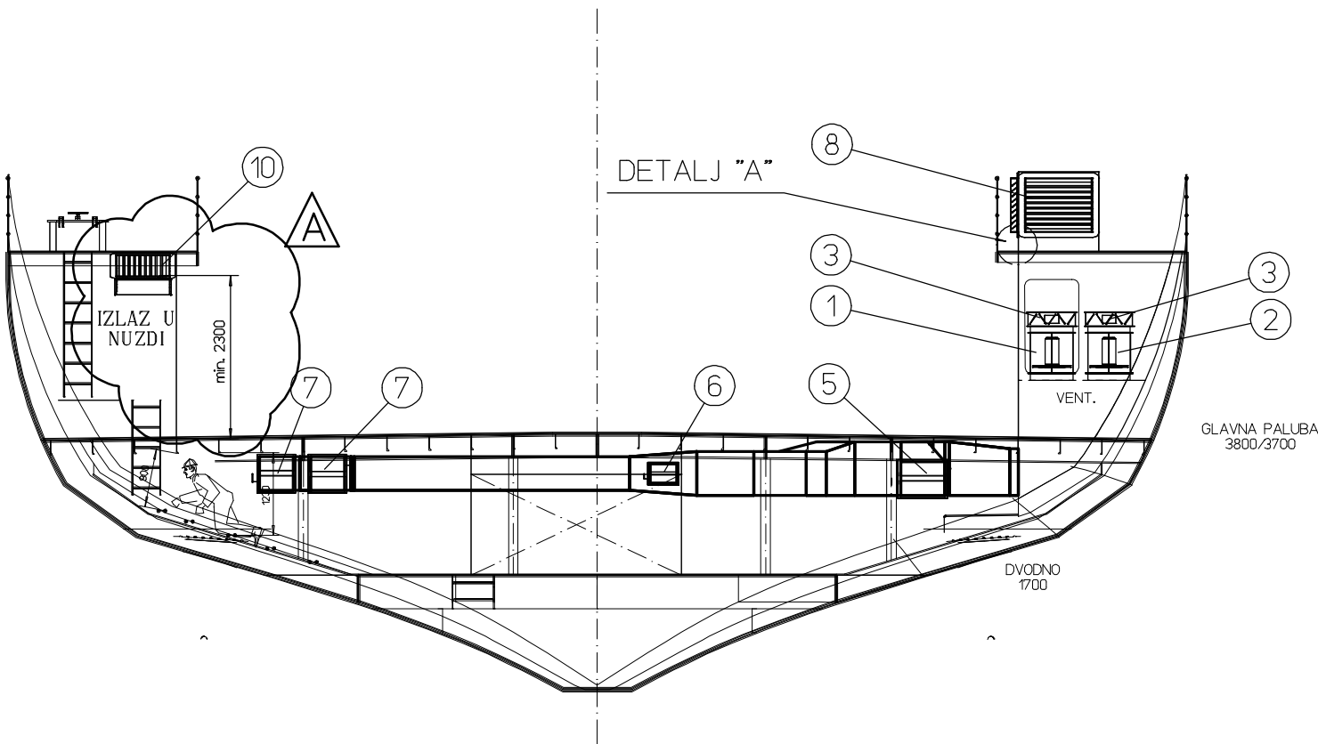
POPREČNI PRESJEK R.16 PREMA KRMU
