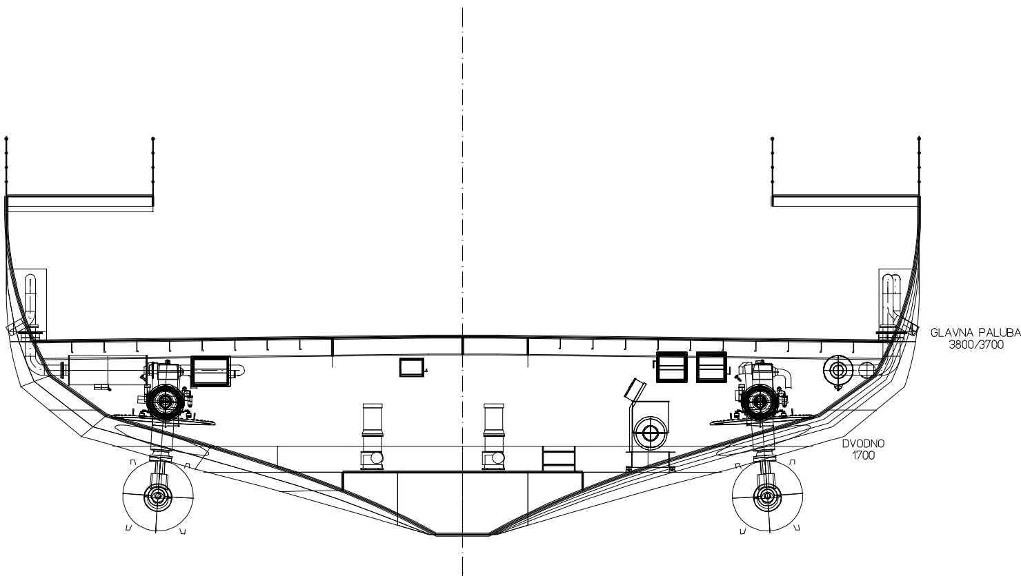
POPREČNI PRESJEK R.16 PREMA PRAMCU
