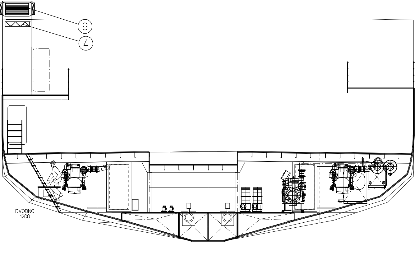
POPREČNI PRESJEK R.22 PREMA PRAMCU
