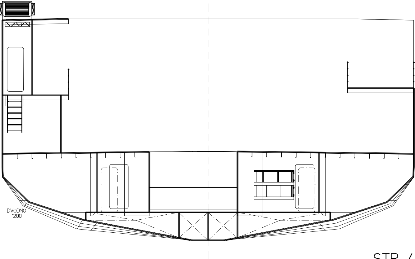
POPREČNI PRESJEK R.28 PREMA PRAMCU
